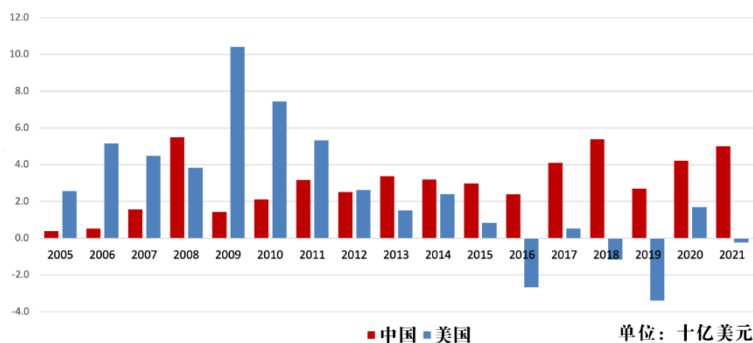
中美对非直接投资（流量）
