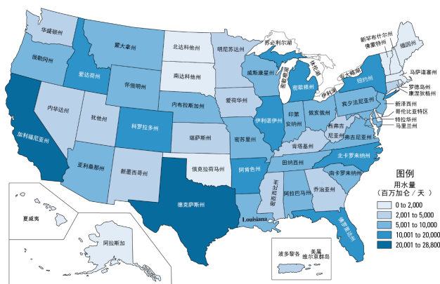
美国各州用水量
